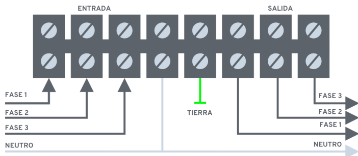
DIAGRAMA CONEXIONES TRIFASICO
